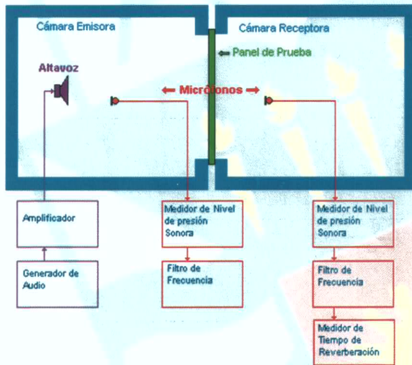
Fig. N°1: Esquema montaje experimental.
