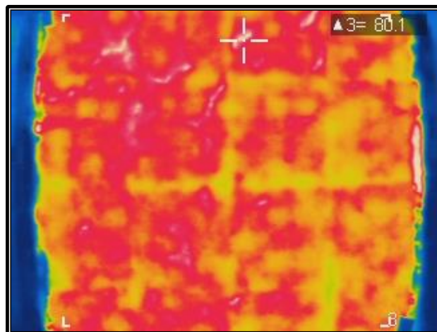
Figura 6.3 Imagen termográfica al término del ensayo
